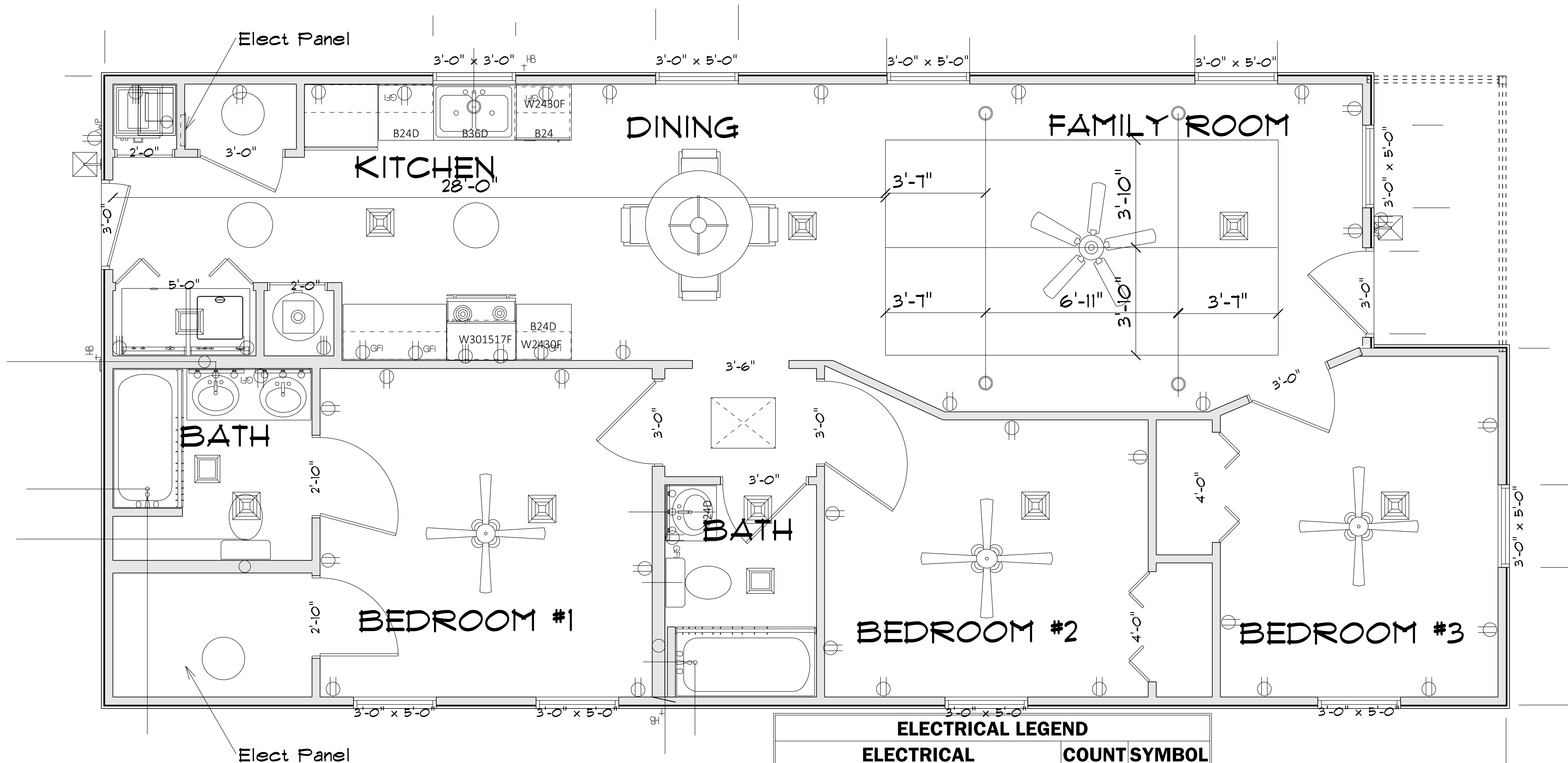
THE SHAWNEE - ELECTRICAL SCALE: 1/2" = 1'-0"
