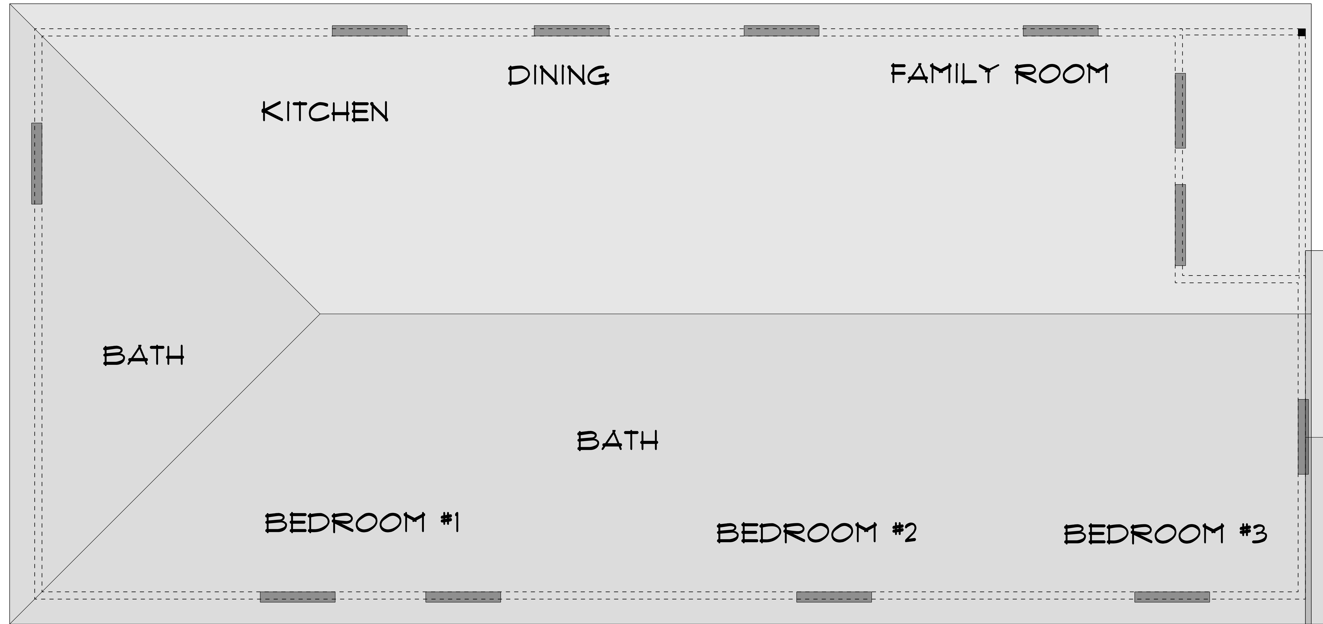
THE SHAWNEE - ROOF SCALE: 1/2" = 1'-0"
