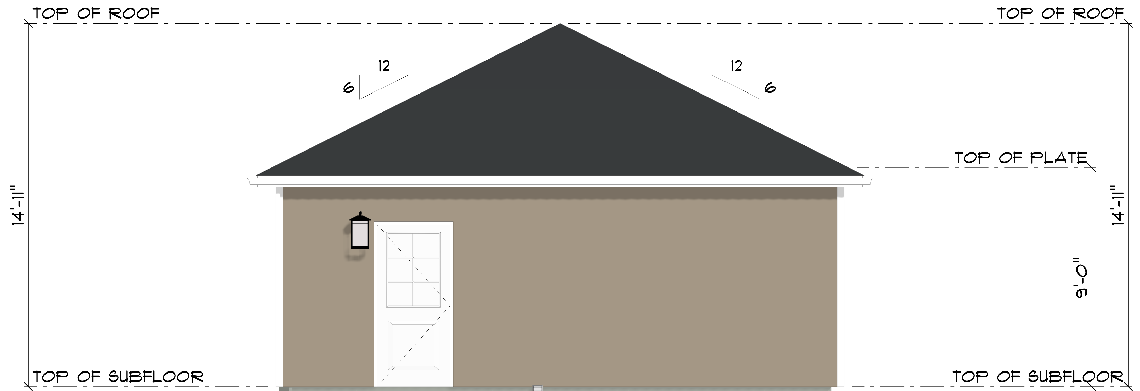
WEST ELEVATION SCALE: 1/2" = 1'-0"
